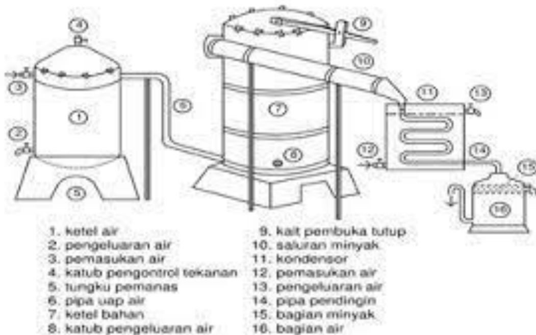
Gambar 2. Model alat pembuatan minyak atsiri secara konsep
