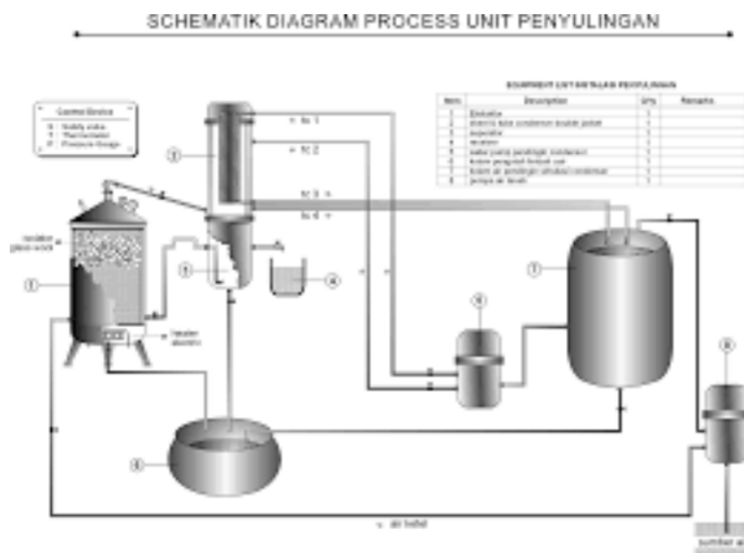
Gambar 1. Konsep skematis Penyulingan Minyak atsiri secara destilasi
