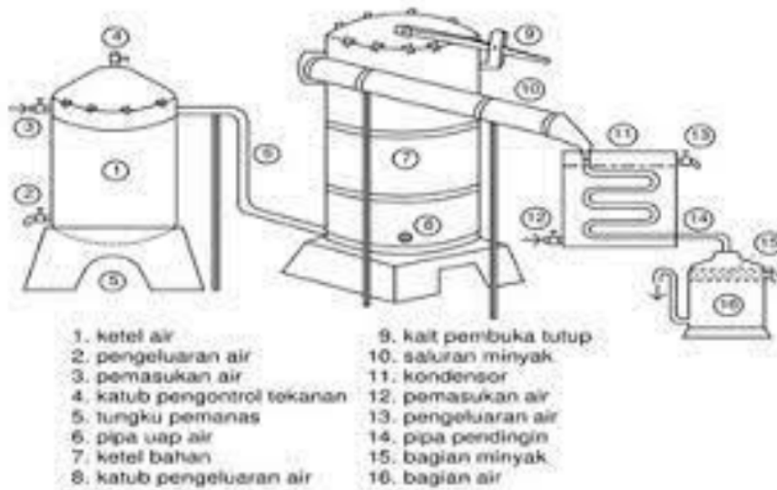
Gambar 2. Model alat pembuatan minyak atsiri secara konsep
