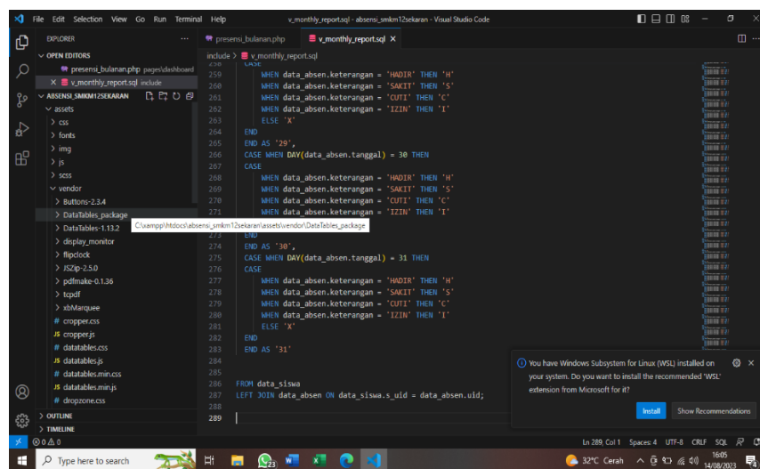
Gambar 4. 11 Visual Code
