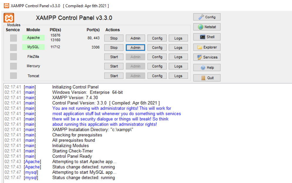
Gambar 2. 8 XAMPP
