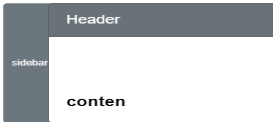
Gambar 4. 6 Rangka Antarmuka
