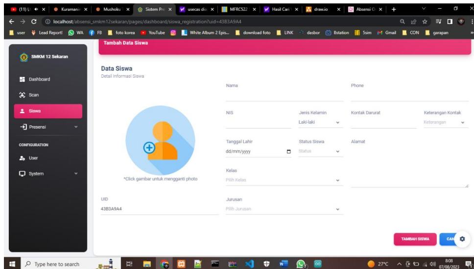
Gambar 4. 16 Tambah Siswa
