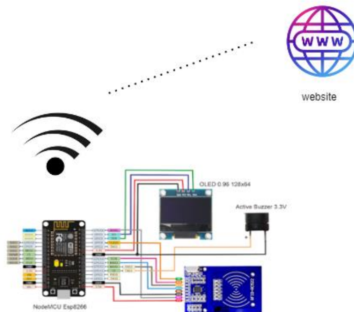
Gambar 4. 1 Skema Rangkaian
