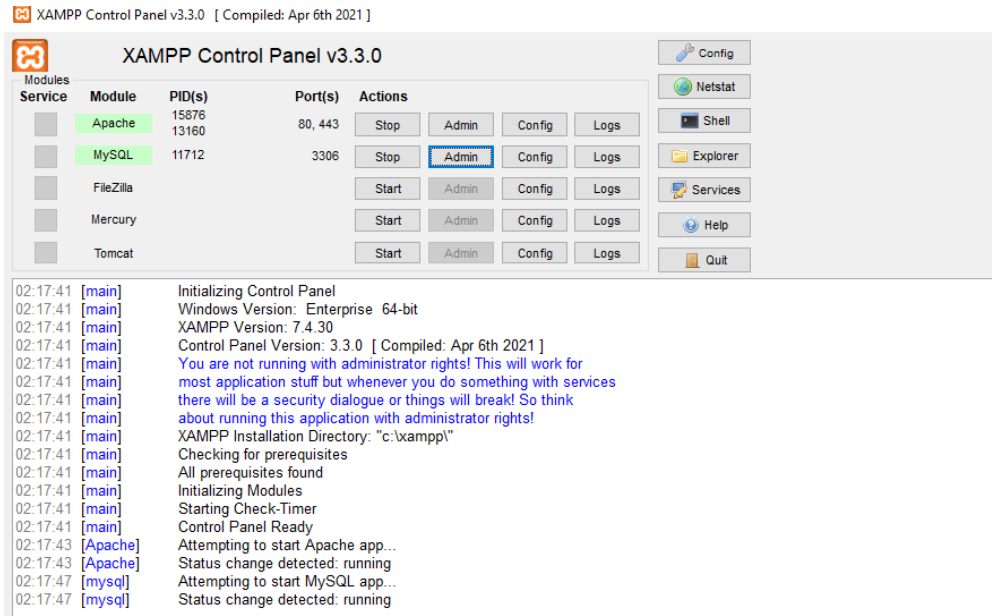
Gambar 4. 10 Xampp
