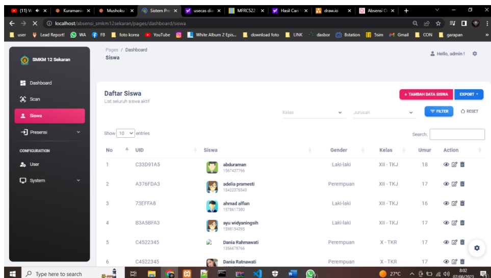
Gambar 4. 17 Data Siswa
