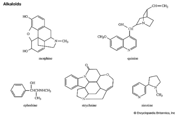
Gambar 1. Struktur Kimia Alkaloid secara umum
