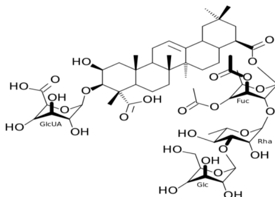
Gambar 4. Stuktur Saponin (steroid)
