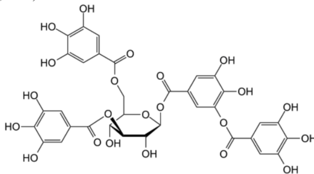
Gambar 2. Struktur Kimia Tanin secara umum
