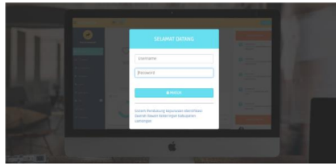
Gambar. 2 Login page
