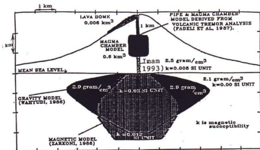
2 Hasil interpretasi bawah permukaan Gunung Merapi dari beberapa macam metode. (Sumber: Suyanto, 2012)
