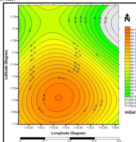
Gambar 4 Kontur Anomali Bouguer Regional dengan pengangkatan 500 meter
