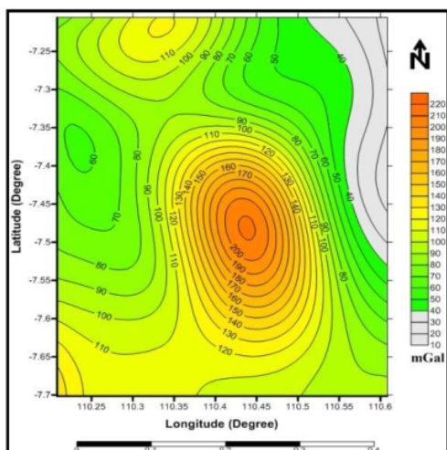
Gambar 3 Kontur Anomali Bouguer Lengkap Gunung Merapi
