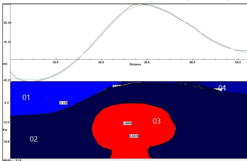
Gambar 8 Pemodelan Bawah Permukaan Lintasan C-D
