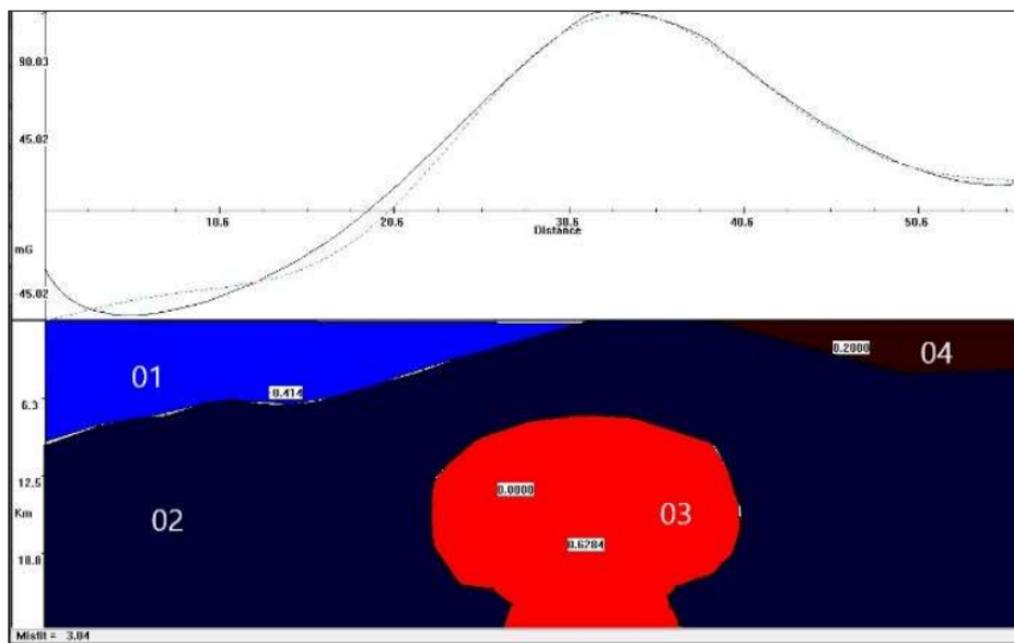
Gambar 9 Pemodelan Bawah Permukaan Lintasan E-F
