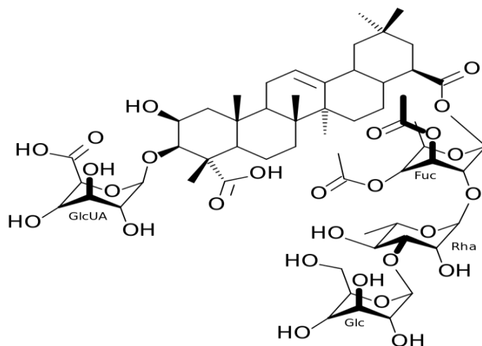
Gambar 4. Struktur Saponin (steroid)
