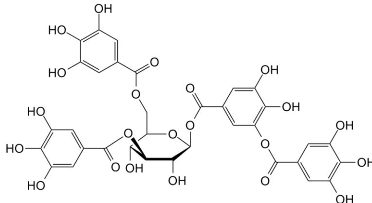
Gambar 2. Struktur Kimia Tanin secara umum
