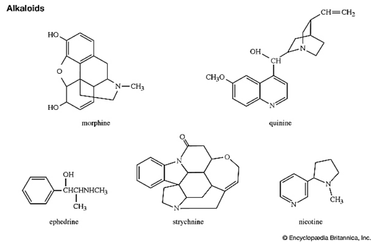
Gambar 1. Struktur Kimia Alkaloid secara umum
